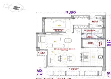
TIPO-04 VIVIENDAS Nº: 15, 16 y 17 PL/ BAJA.
