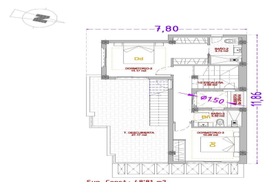
TIPO-04 VIVIENDAS Nº: 15, 16 y 17 PL/ PRIMERA.
